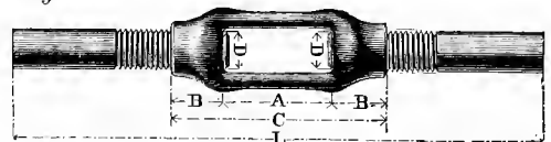
Fig. 3727a. PATENT TURNBUCKLE, R. AND L.
